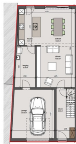
Voorbeelden plattegrond met inpandige garage. De maatvoering kijkt af van de kavels. Deze voorbeelden zijn daarom puur ter inspiratie.
